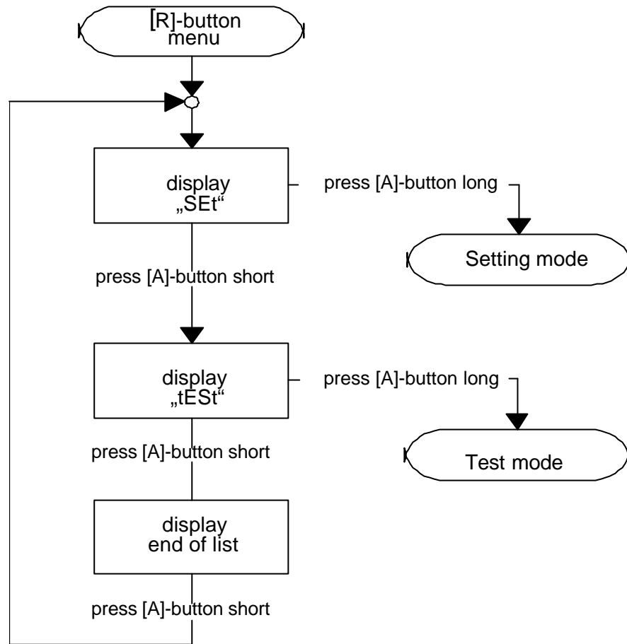
Fig. 7 R-button menu
